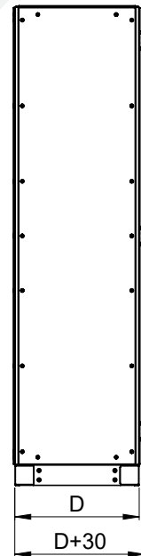
YAN GÖRÜŞÜ
