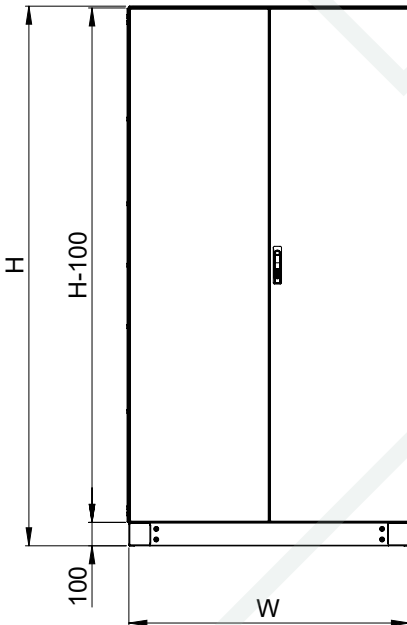
ÖN GÖRÜŞÜ
