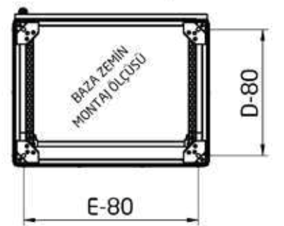
ALT GÖRÜNÜŞ
