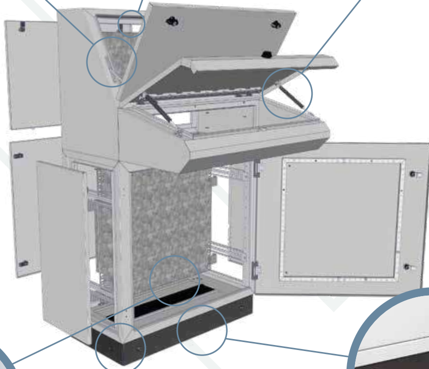
Amortisör Tutucu
