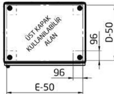
ÜST GÖRÜNÜŞ
