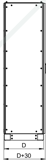
YAN GÖRÜNÜŞ
